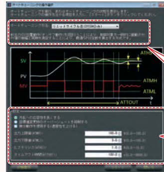
〈オートチューニング設定〉
