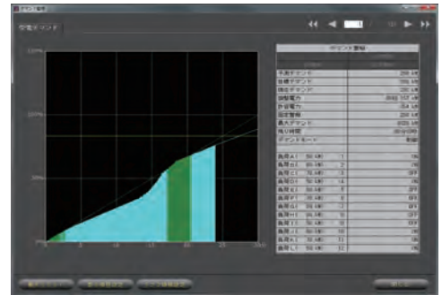
〈デマンド監視・制御〉
